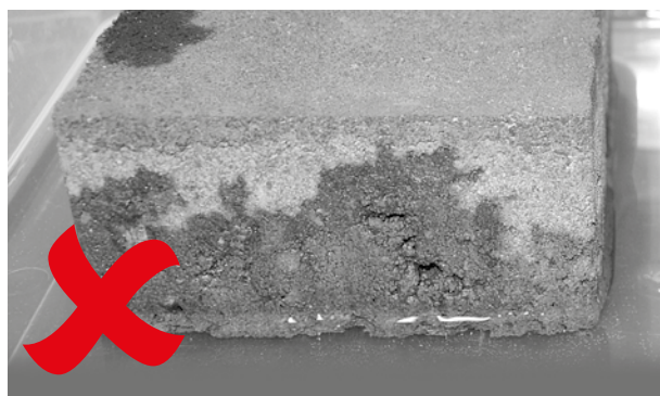
Настилка без хидрофобизираща добавка
