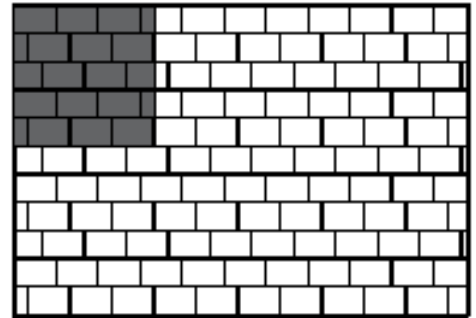
Растер 8 30x20x8cm - 16.67 броя Разход на м 2
