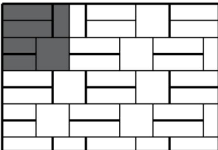
Растер 3 50x50x8cm - 1,50 броя 75x25x8cm - 3,34 броя Разход на m 2
