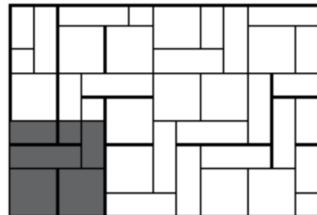
Растер 4 50x50x8cm - 2 броя 75x25x8cm - 2,67 броя Разход на m 2
