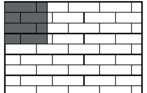
Растер 12 75x25x8cm - 5.34 броя Разход на м 2
