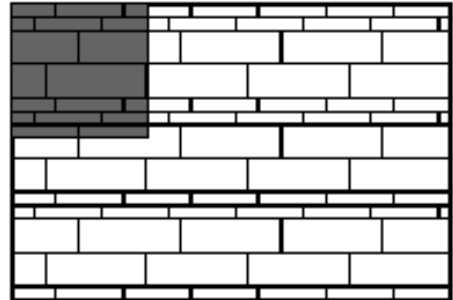
Растер 2 75x25x8cm - 3,21 броя 50x10x8cm - 8 броя Разход на m 2
