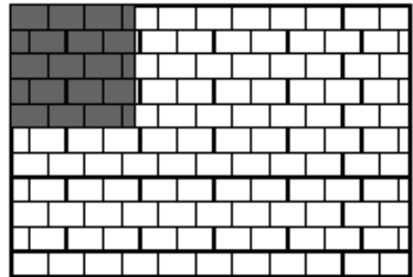
Растер 6 30x20x8cm - 16,71 броя Разход на m 2
