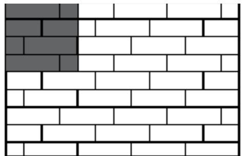
Растер 10 75x25x8cm - 5.34 броя Разход на м 2
