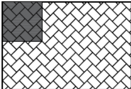
Растер 9 30x20x8cm - 16.65 броя Разход на м 2
