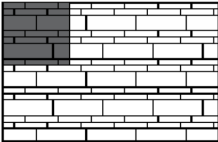
Растер 1 75x25x8cm - 2,67 броя 50x10x8cm - 10 броя Разход на m 2
